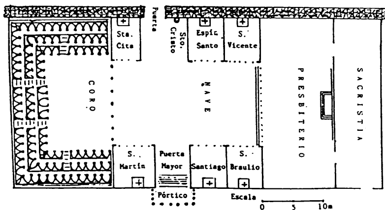
Planta de Santa María la Mayor.
