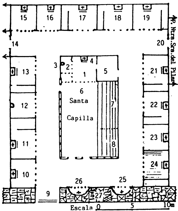
Claustro y capillas claustrales.
